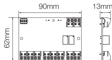
Dimensioni
