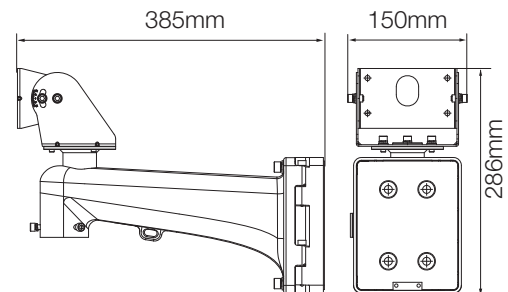
Dimensioni
