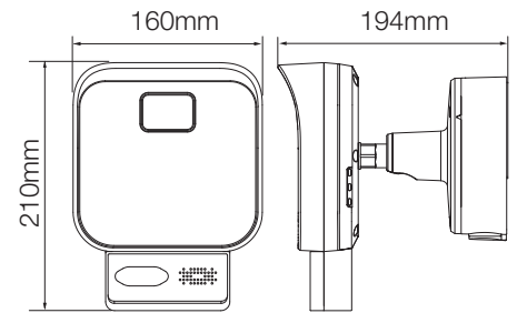
Dimensioni
