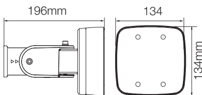
Dimensioni
